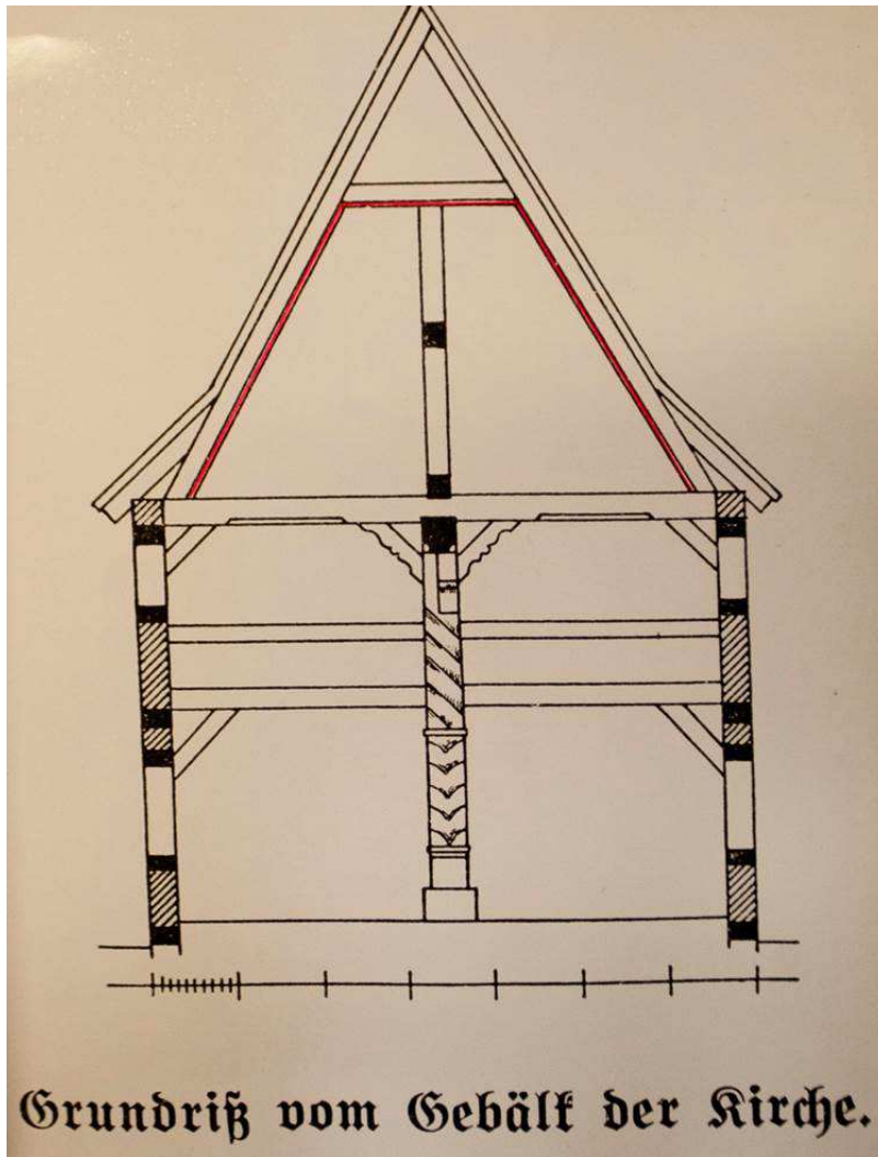
Historischer Querschnitt Einstützenraum-Konstruktion
